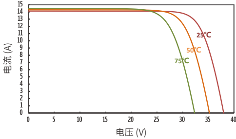
JT420SEt 不同温度下的IV曲线
