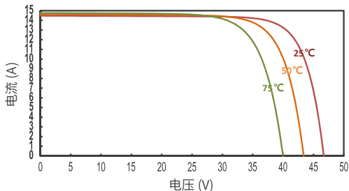
JT530Sft 不同温度下的IV曲线
